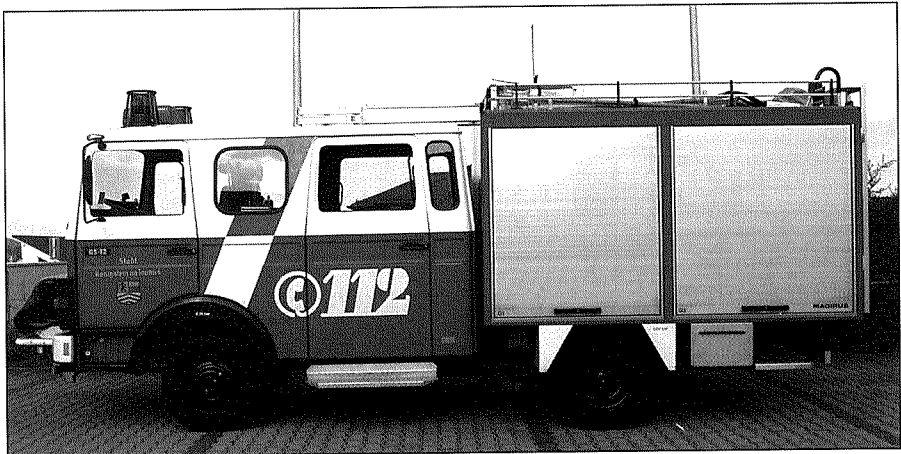
LF 8. Iveco Magirus, zul. Gesamtgewicht 6,9t, 114 PS, Baujahr: 1990. Löschgruppenfahrzeug, Feuerlöschkreiselpumpe 8/8, Tragkraftspritze 8/8, Besatzung: 1/8. Nachrückendes Löschfahrzeug bei Brandeinsätzen, einziges Königsteiner Löschfahrzeug, das in die Altstadt fahren kann, erstes Fahrzeug bei Wassereintrüben, Übungsfahrzeug der Jugendfeuerwehr. Ausrüstung: 4 Preßluftatmer, Löschausrüstung, 4-teilige Steckleiter (8,4m), Tauchpumpen, Industriesauger. Gefahrene Einsätze im Jahr 2000: 22
