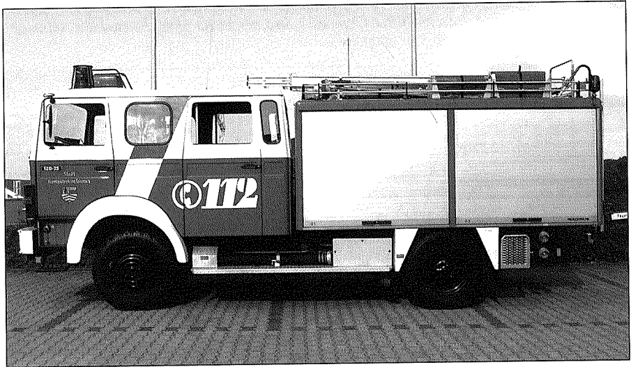
TLF 16/25. Iveco Magirus, zul. Gesamtgewicht 12t, 256 PS, Allrad, ABS, Schleuderketten, Baujahr 1987. Tanklöschfahrzeug, 2500l Wassertank, 100l Schaummitteltank, Feuerlöschkreiselpumpe 16/8 mit Hochdruckteil, Besatzung: 1/5. Erstes Fahrzeug im Löschzug, zweites Fahrzeug bei Verkehrsunfällen. Ausrüstung: 30 m Schnellangriff, 80m Hochdruckschnellangriff (bis 40 bar), Schaumschnellangriff, Dachmonitor, 4 Preßluftatmer davon 2 im Mannschaftsraum, Löschausrüstung, 4-teilige Steckleiter (8,4m), hydraulische Rettungsschere mit Handbetrieb, Sprungretter, Notfallkoffer, Einsatzpläne Gefabrene Einsätze im Jahr 2000: 37
